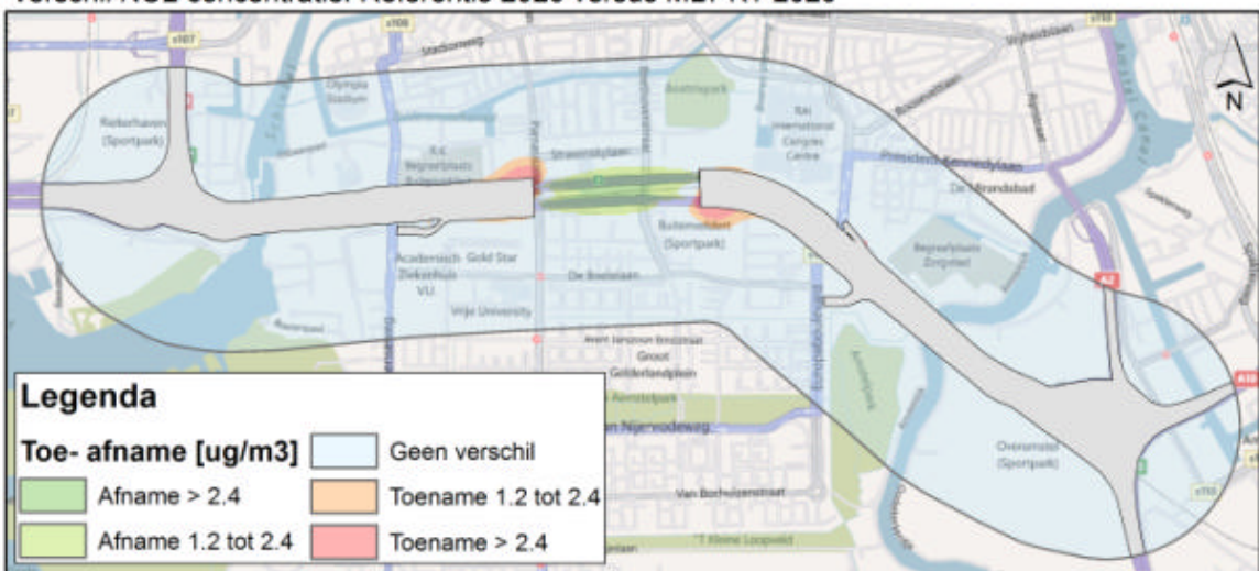
figuur 9.6 Verschilkaart concentraties NO 2 tussen de referentiesituatie 2020 en de MLT (boven lange tunnel, onder korte tunnelvariant)
