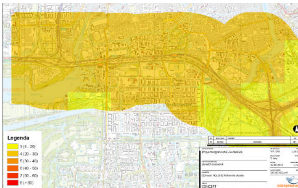
figuur 14.4 Luchtkwaliteit NO 2 referentie
