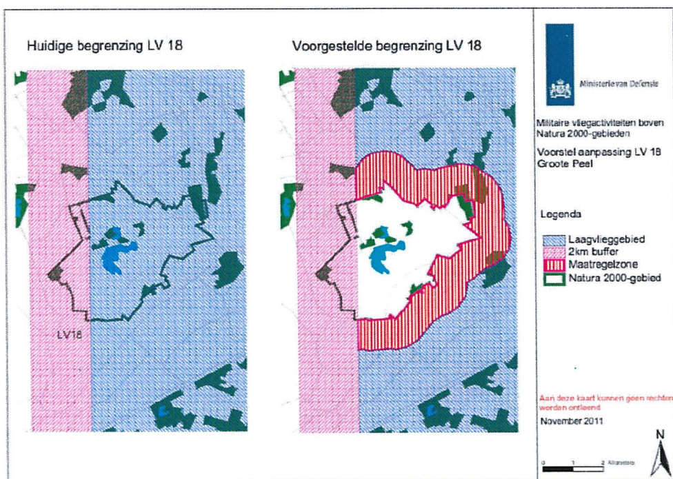
Figuur 6.1: Laagvlieggebied 18 (Peel) voorgestelde grenscorrectie in het kader van de maatregel voor Natura 2000 gebied Groote Peel.
