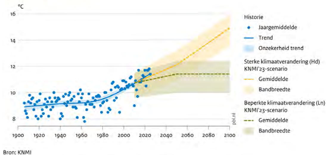
Figuur 2.1 Temperatuur in Nederland
