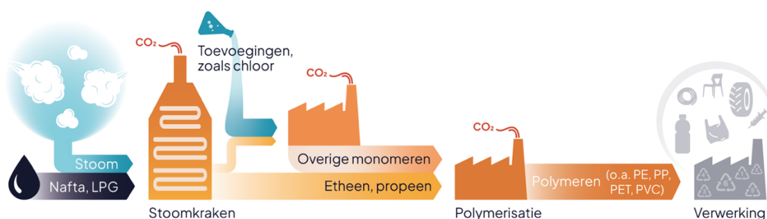
Figuur 8. Schematisch overzicht van de productie van kunststoffen. Grondstof- en energiestromen zijn versimpeld ten opzichte van de werkelijkheid.
