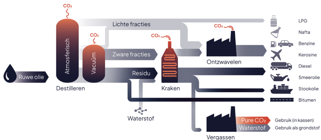
Figuur 7. Schematisch overzicht van het raffinageproces. Grondstof- en energiestromen zijn versimpeld ten opzichte van de werkelijkheid. Ook zijn mogelijke (na)bewerkingsstappen weggelaten of samengevoegd om de leesbaarheid te vergroten.
