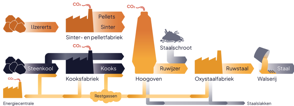
Figuur 6. Schematisch overzicht van staalproductie volgens het BF-BOF-proces. Dit is het proces waarmee Tata Steel nu in Nederland staal maakt. Grondstof- en energiestromen zijn versimpeld ten opzichte van de werkelijkheid.
