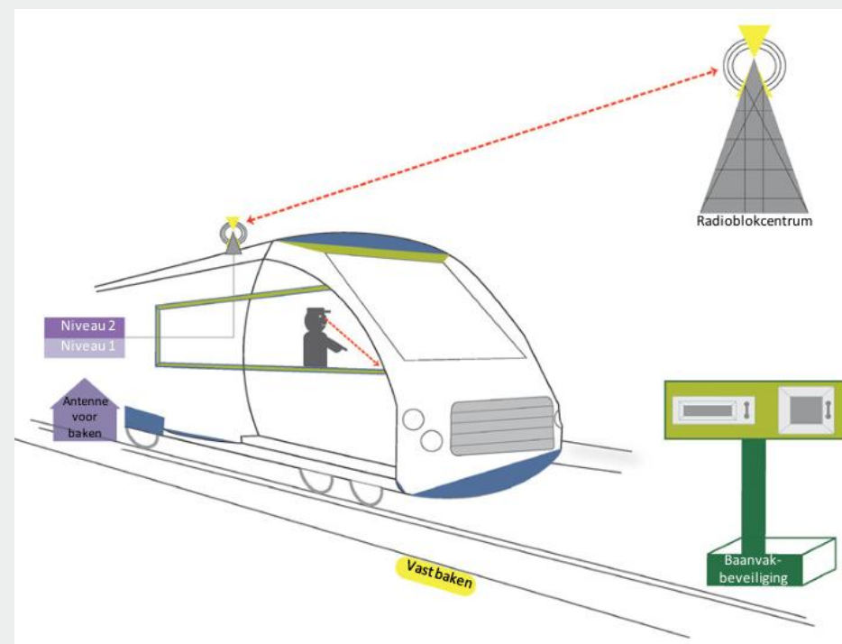
Figuur 1 van SR 13/2017 - de werking van het Europees beheersysteem voor het spoorverkeer (ERTMS) waar het treinbesturingssysteem (ECTS) onderdeel van uitmaakt (bladzijde 14) en kader 6.4 van het jaarverslag 2025 van de ERK
