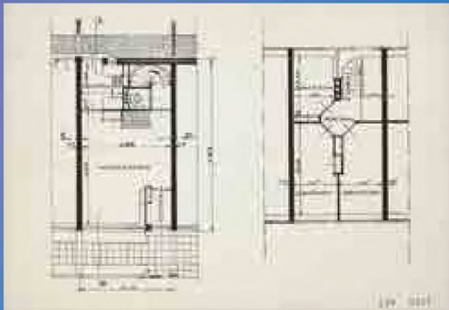
Afbeelding 20. Plattegrond van woningen in de wijk Kiefhoek gebouwd naar het ontwerp van de architect J.J.P. Oud. Bron: Rijksvoorlichtingsdienst (RVD), bestandnr. I30-0457, Nationaal Archief.
